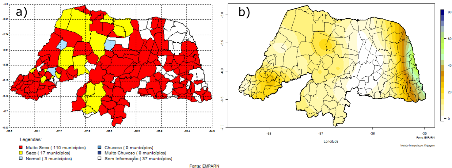
Figura 1: (a) Classificação climática das chuvas nos municípios, e (b) Precipitação acumulada no mês de Junho.
